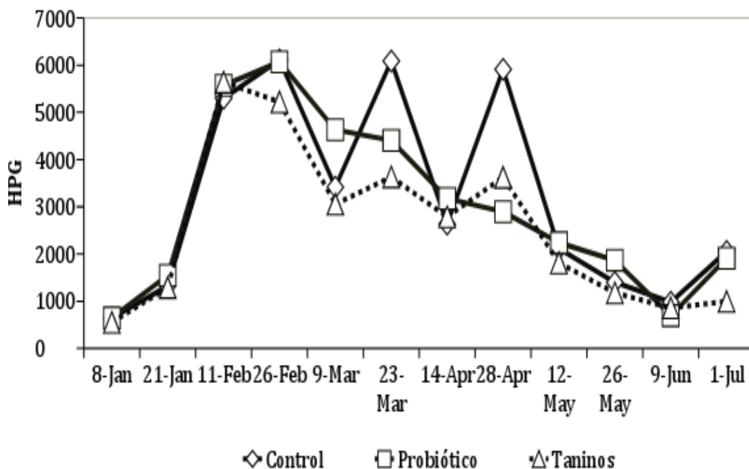
Figura 4. Evolución promedio de los conteos de huevos por gramo (HPG) de materia fecal de los corderos sometidos a los tres tratamientos, durante el período experimental (enero-junio 2016).
