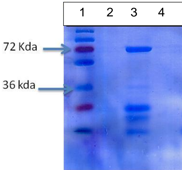
Figura 7. SDS PAGE 12% del 2 cromatograma de purificación de Bm86uy-r. (figura 6). 1) Peso molecular, 2) tubo 7 de colecta pre-elusión de la proteína; 3) tubo 8 donde está Bm86uy-r eluida de la columna por 500mM de Imidazol; 4) tubo 9 pos elución de la Bm86uy-r indicando que no queda nada pegado a la misma.
