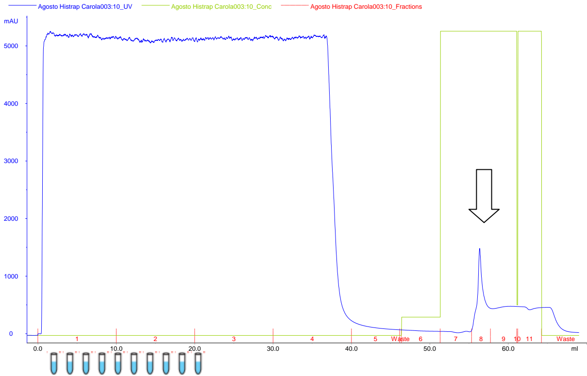
Figura 6. Segundo Cromatograma de la proteína recombinante Bm86uy-r por columna de Histrap purificada, utilizando mayor volumen de cultivo. El pico de salida de la proteína recombinante Bm86uy-r se observa en el pico indicado por la flecha eluida (desprendida por la columna) con Imidazol 500 mM.
