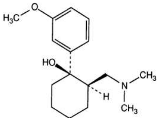
Figura 3: Molécula Tramadol
